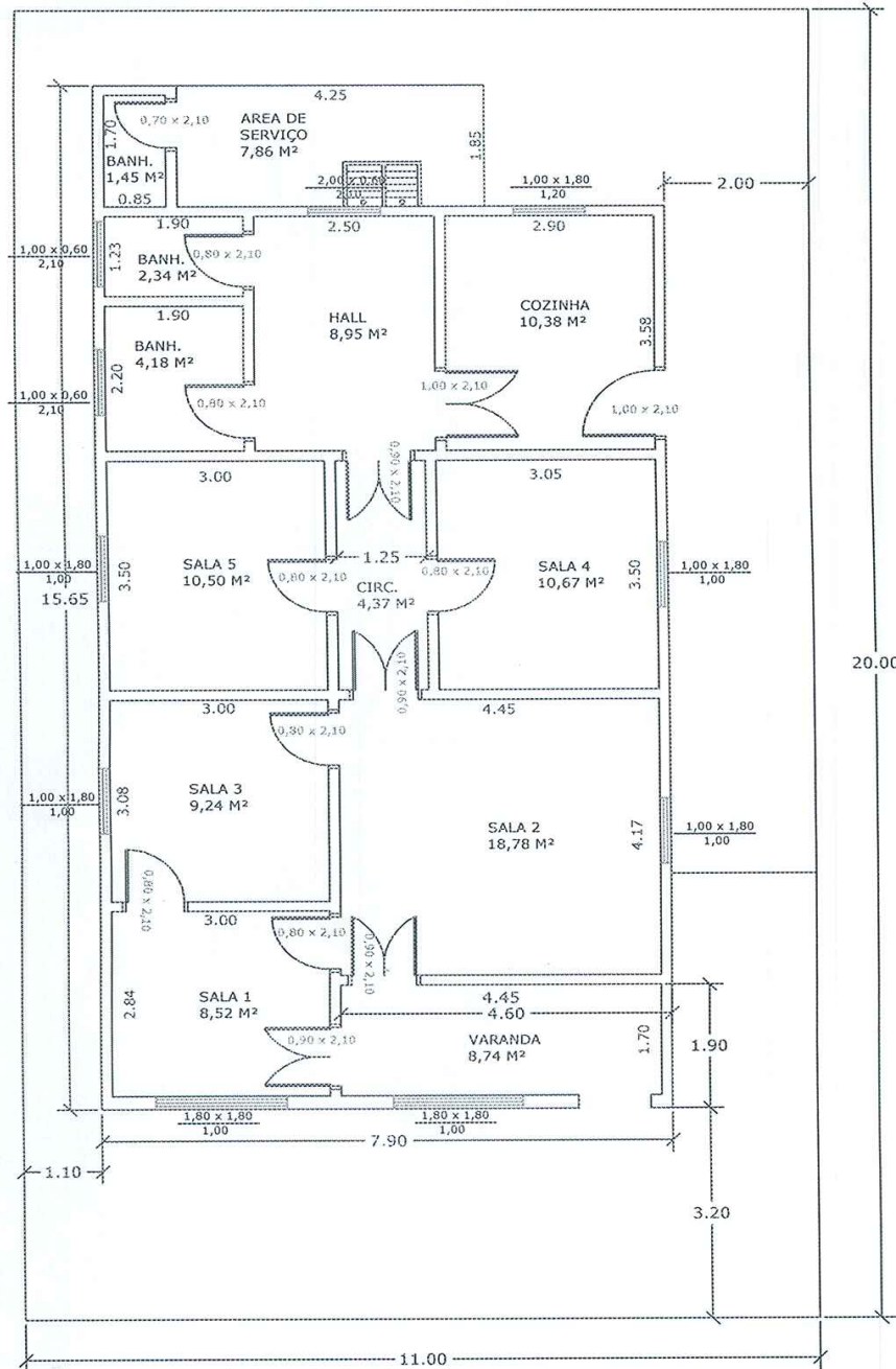
PLANTA BAIXA ESCALA 1:100
