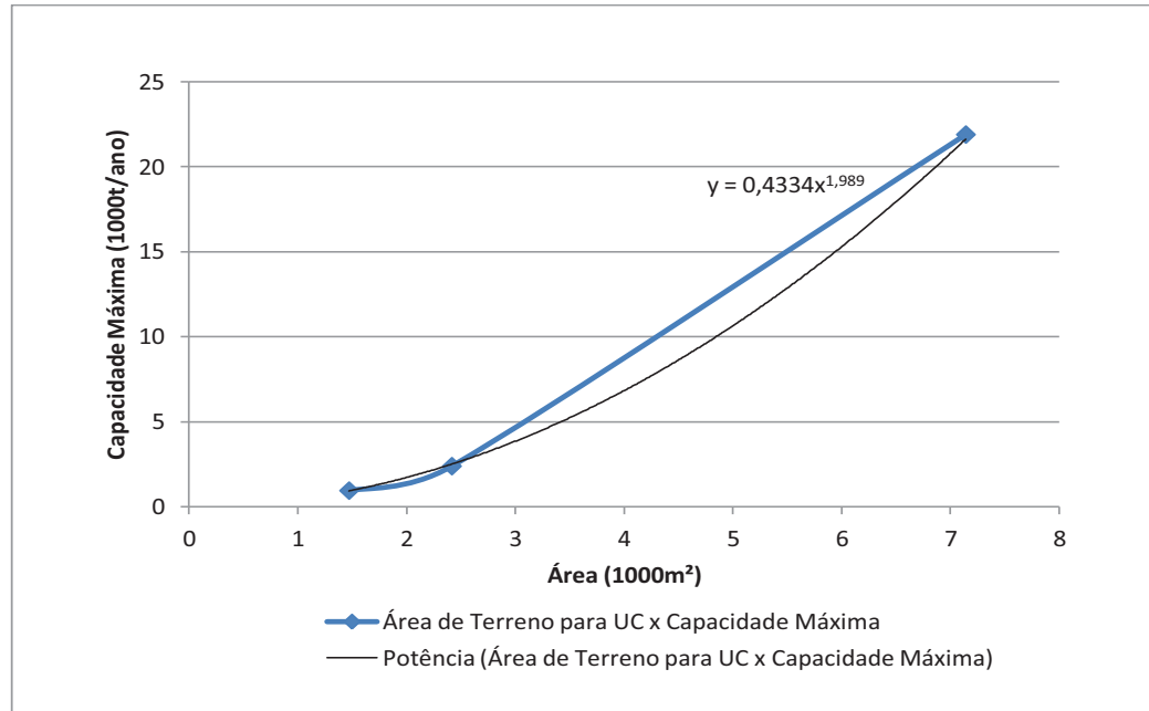
Gráfico 8.2 – Variação da área do terreno da Usina de Compostagem (UC) em função da capacidade
