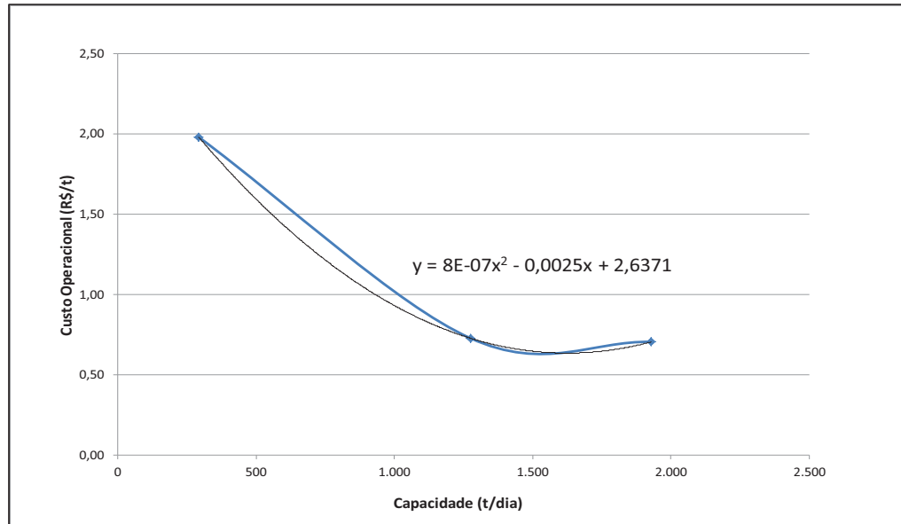
Gráfico 9.6 – Variação do custo operacional de RCC em função da capacidade
