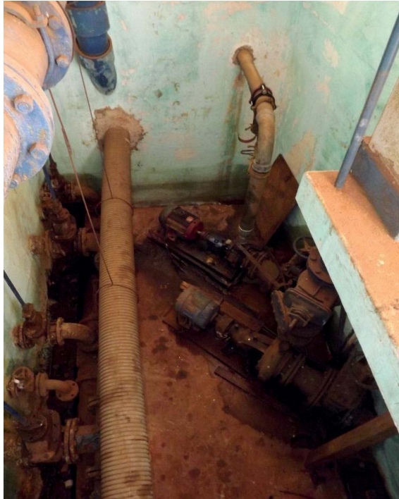
Foto 3.47 – Conjuntos motobomba para retrolavagem e recalque para REL Vila Nova
