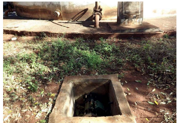
Foto 3.33 – Detalhe do macromedidor instalado na saída do RAP Redona
