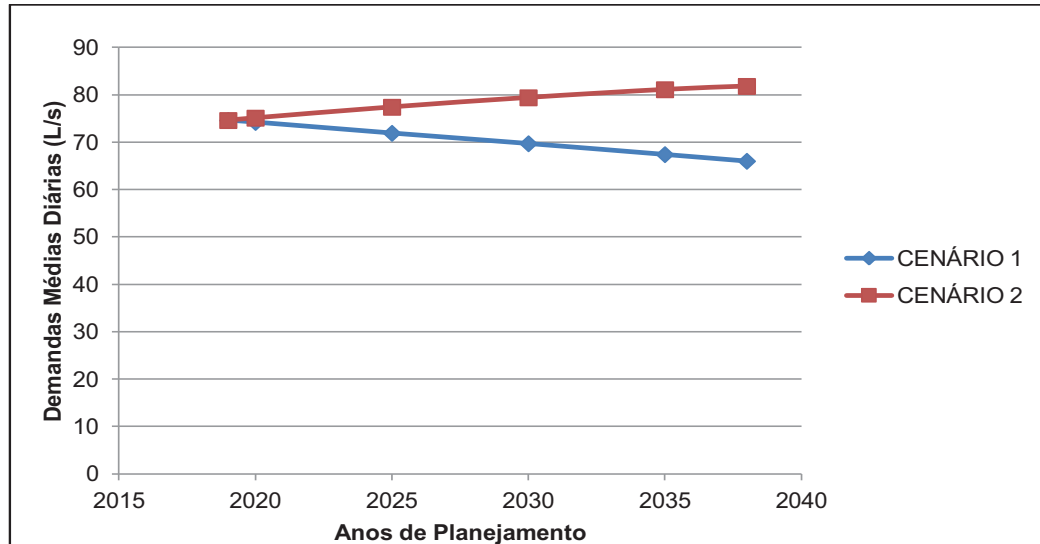
Gráfico 6.2 - Comparação de Demandas - Períodos Quinquenais - 2019 a 2038 – Viradouro
