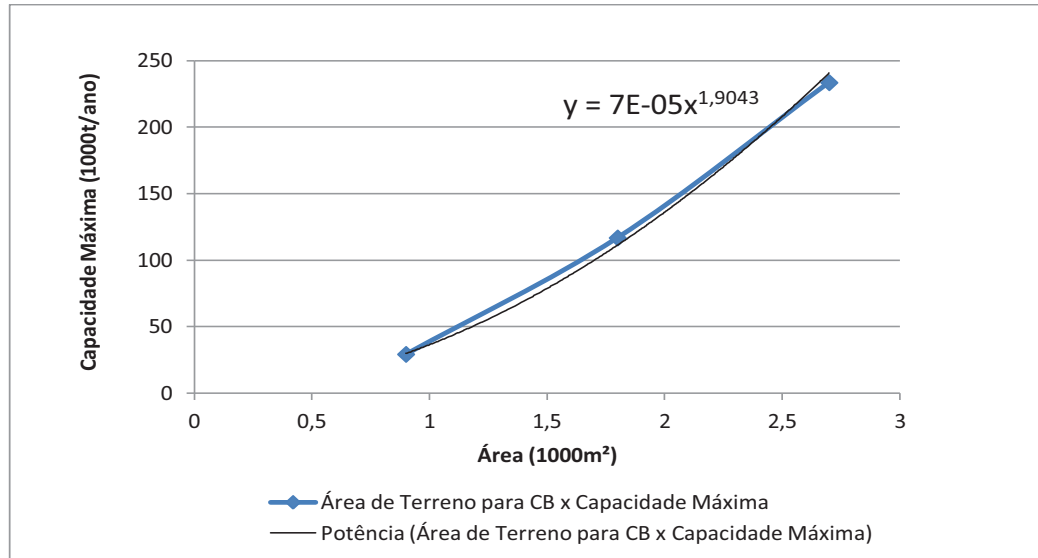
Gráfico 8.4 – Variação da área do terreno da Central de Britagem (CB) em função da capacidade
