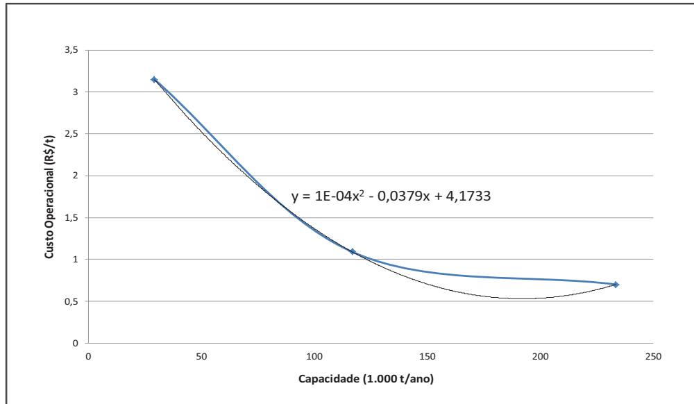
Gráfico 9.4 – Variação do custo operacional da CB em função da capacidade
