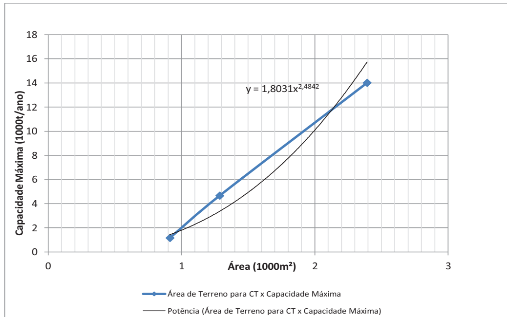
Gráfico 8.1 – Variação da área do terreno da Central de Triagem (CT) em função da capacidade
