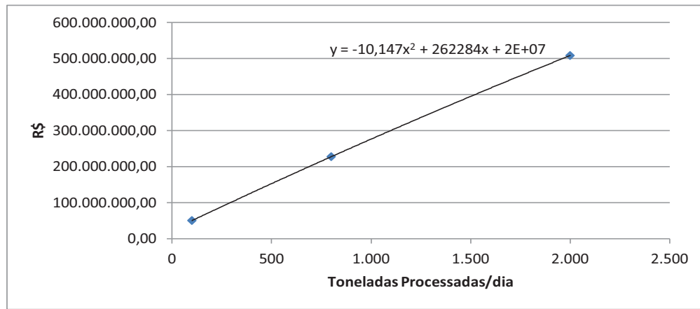
Gráfico 9.2 – Variação do custo operacional do ATS em função da quantidade de resíduos processados por dia
