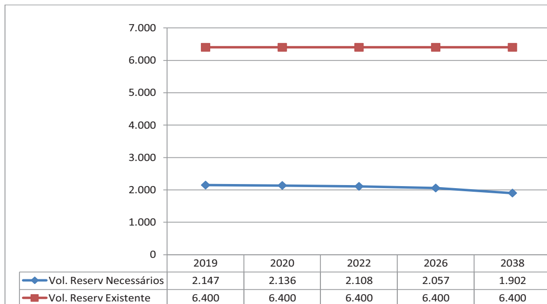
Gráfico 4.5 – Volumes de Reservação Necessários (m³) x Volume de Reservação Existente (m³) x Anos de Planejamento
