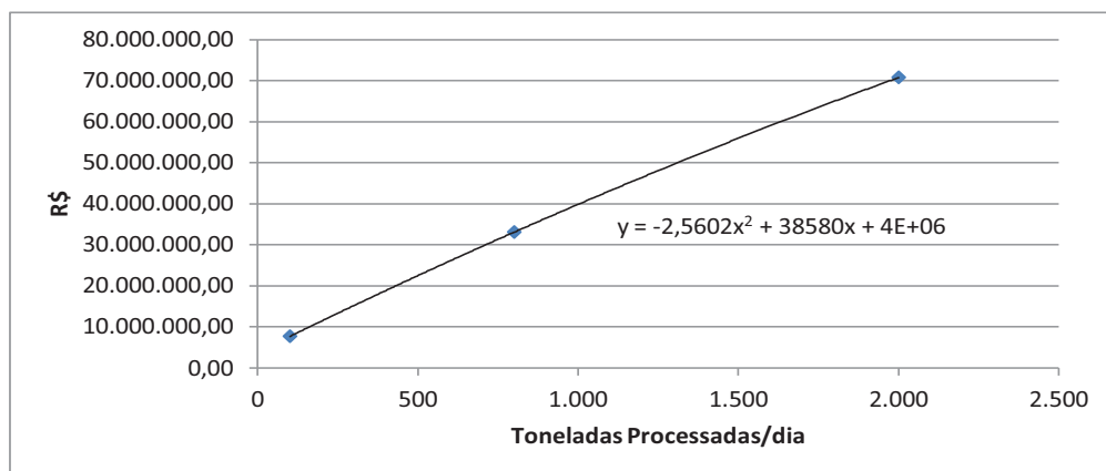
Gráfico 9.1 – Variação do custo de implantação do ATS em função da quantidade de resíduos processados por dia
