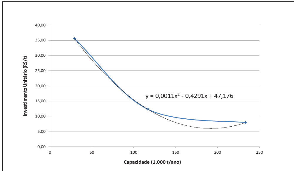
Gráfico 9.3 – Variação do custo de implantação da CB em função da capacidade
