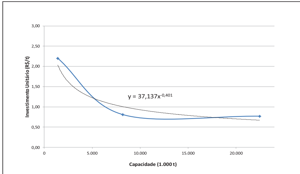
Gráfico 9.5 – Variação do custo da implantação do ARCC em função da capacidade
